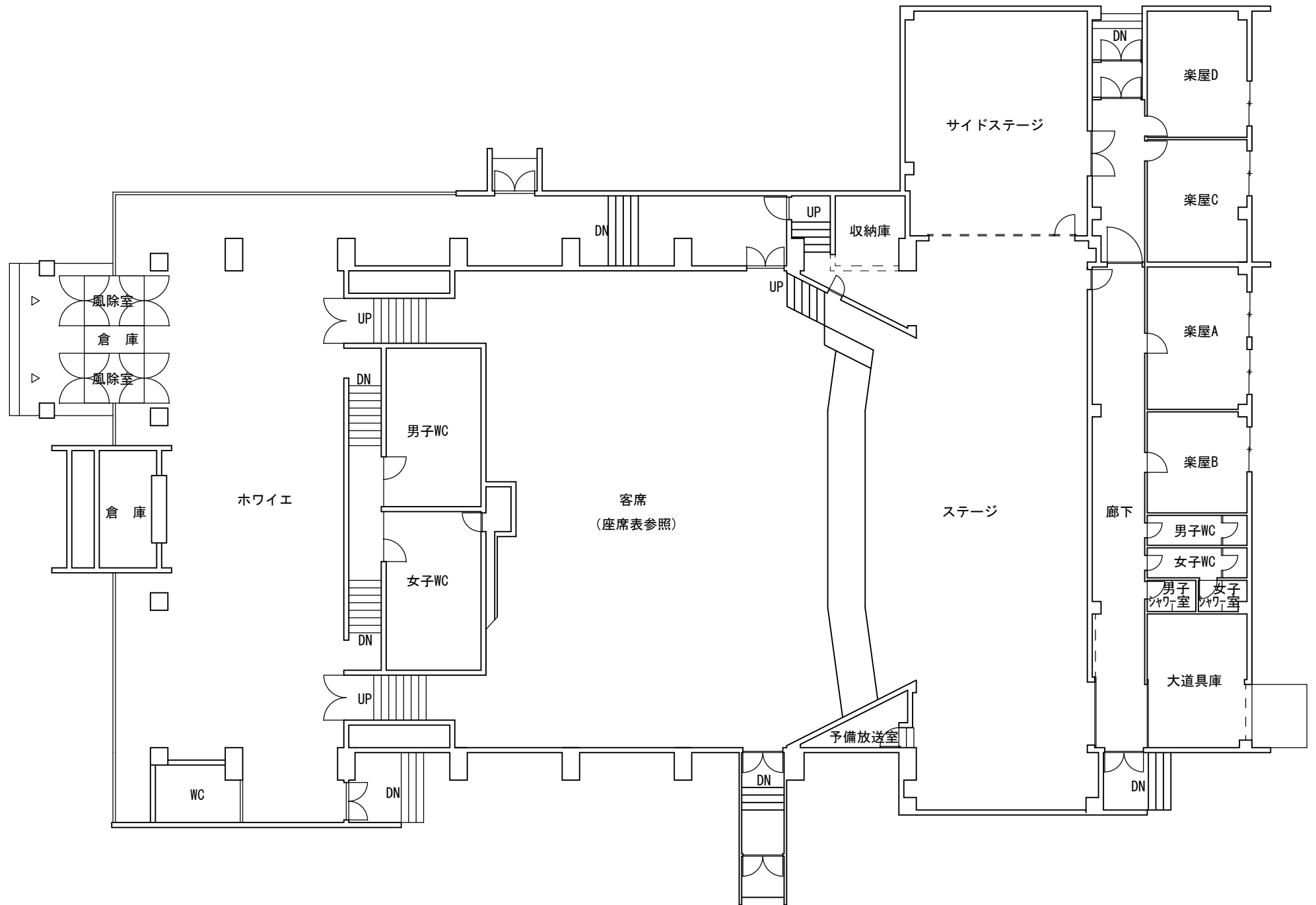
市民会館 1階平面図 S:1/200
